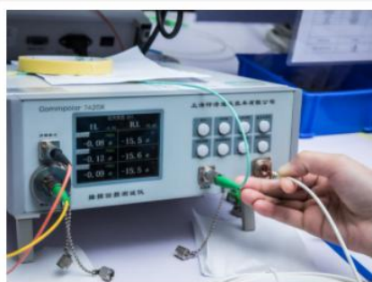
IL/RL test
